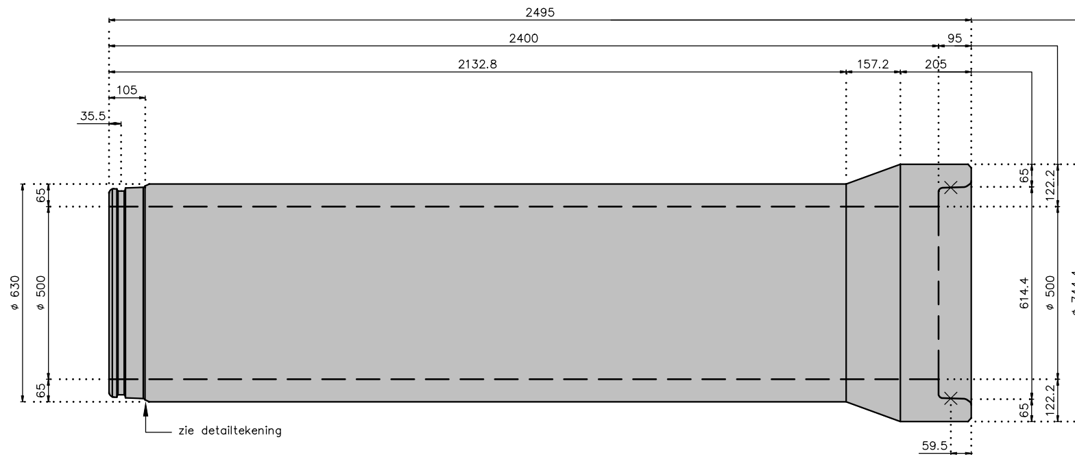
LANGSAANZICHT
